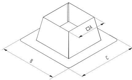
Dachdurchführung Flachdach 0°-10° Solin de toit plat 0°-10°
